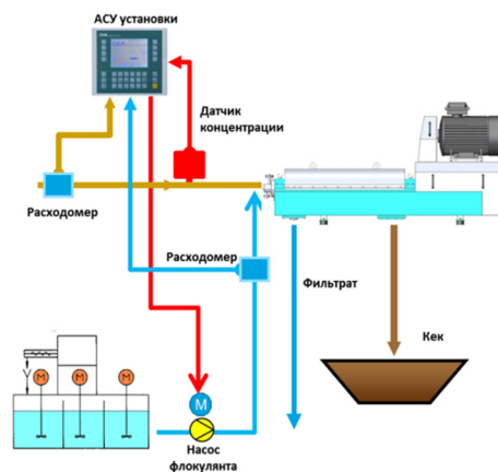
Рис.7. Схема системы автоматического дозирования флокулянта.
