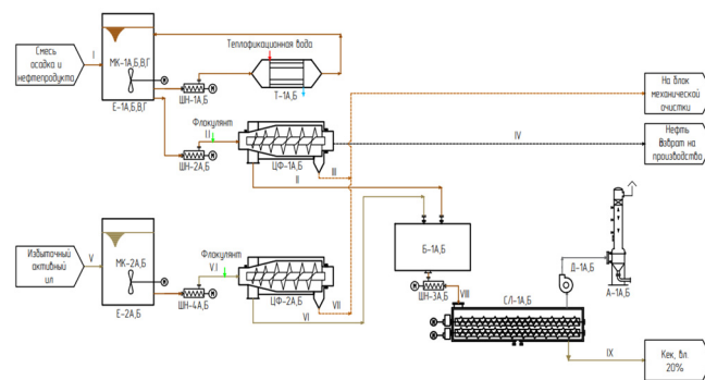
Рисунок 1 – Принципиальная технологическая схема утилизации нефтесодержащих отходов.
