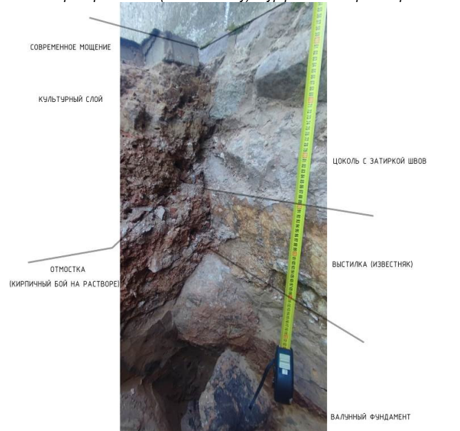
Рис. 3. Ортофотоплан (вид на стену) Шурфа №2 северного фасада.
