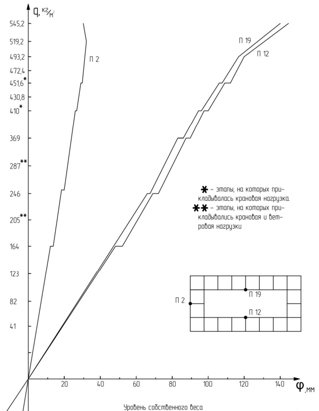
Рис. 3. Графики прогиба конструкции
