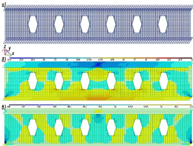
Рис. 7. К расчету стальной предварительно напряженной балки Б4 с перфорацией стенки: а – конечно-элементная модель балки Б4; б – мозаика нормальных напряжений N_x ( \text{kH}/\text{m}^2 ) балки Б4; в – мозаика нормальных напряжений N_y ( \text{kH}/\text{m}^2 ) балки Б4
