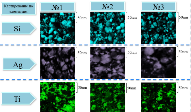
Рис. 2. ПЭМ-фотографии по элементам трех разных по соотношениям нанокompозитов
