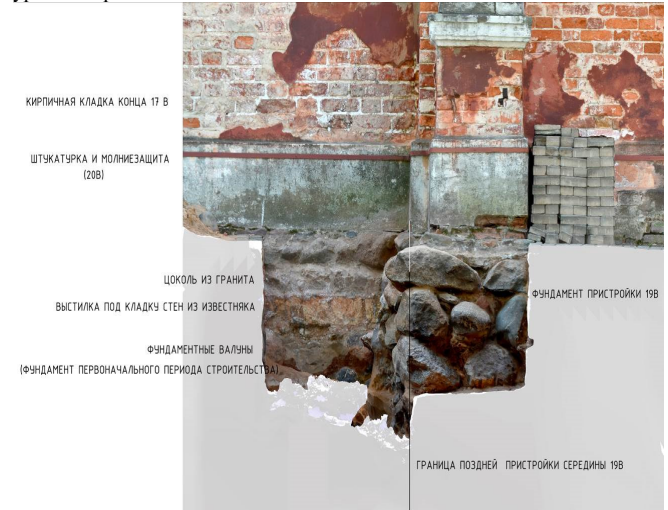
Рис. 3. Ортофотоплан (вид на стену) Шурфа №2 северного фасада.
