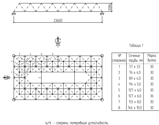
Рис. 1. Структурная конструкция с неполной решеткой а) б)
