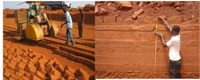
Рис. 3 – Виды карьера Дано: распил блоков и описание забоя
