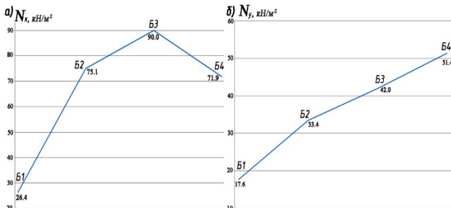
Рис. 8. Величины максимальных нормальных напряжений в балках Б1 – Б4: а – напряжения N_x , \text{kH}/\text{m}^2 ; б – напряжения N_y , \text{kH}/\text{m}^2
