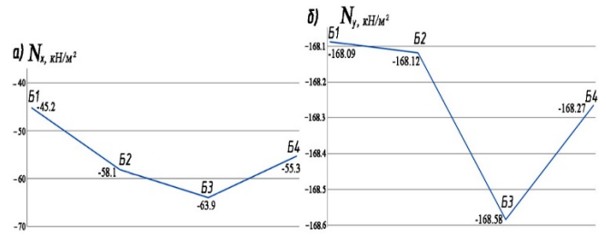
Рис. 9. Величины минимальных нормальных напряжений в балках Б1 – Б4: а – напряжения N_x , \text{kH}/\text{m}^2 ; б – напряжения N_y , \text{kH}/\text{m}^2
