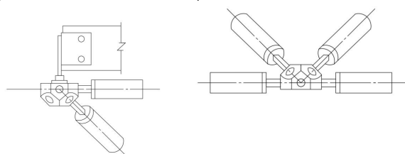
Рис. 2. Типовые решения узлов верхнего а) и нижнего б) поясов
